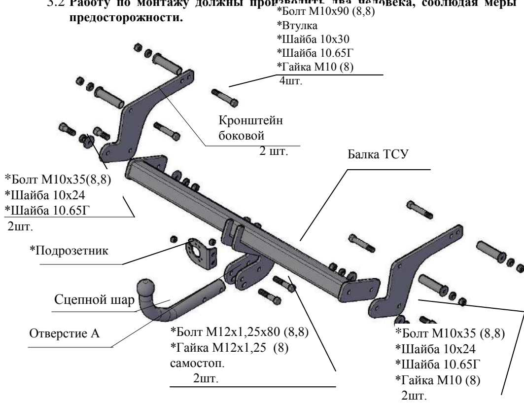
Рис.1 Тягово-сцепное устройство ТСУ 9041.01.
